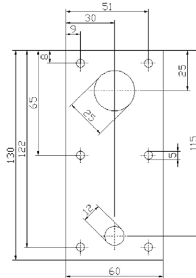
montažna ploča DN25 E-2604260
