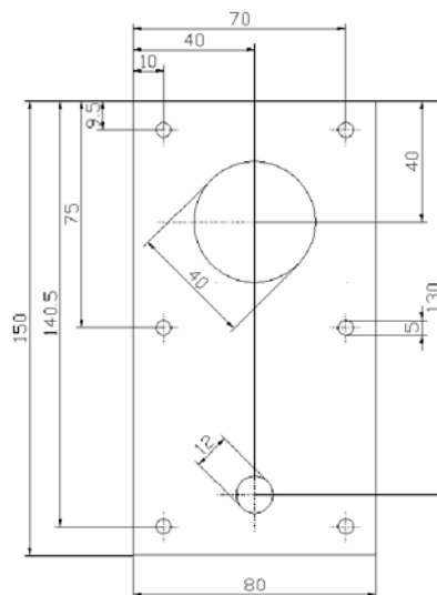
montažna ploča DN40 E-2604410
