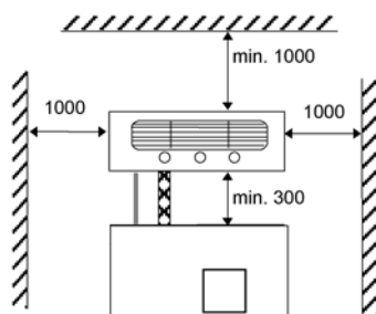
Montaža na zid - pogled sa prednje strane
