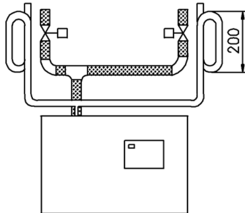
Montaža solenoidnog ventila za paru
